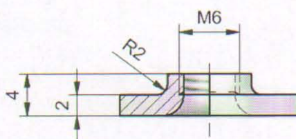
Presek A-A ( 2 : 1 )
