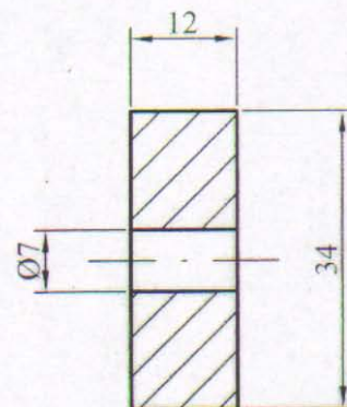
PRESEK „A-A“:
