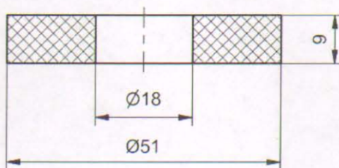
Presek A-A ( 1 : 1 )
