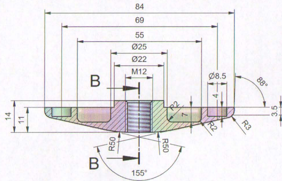
A-A (1:1)
