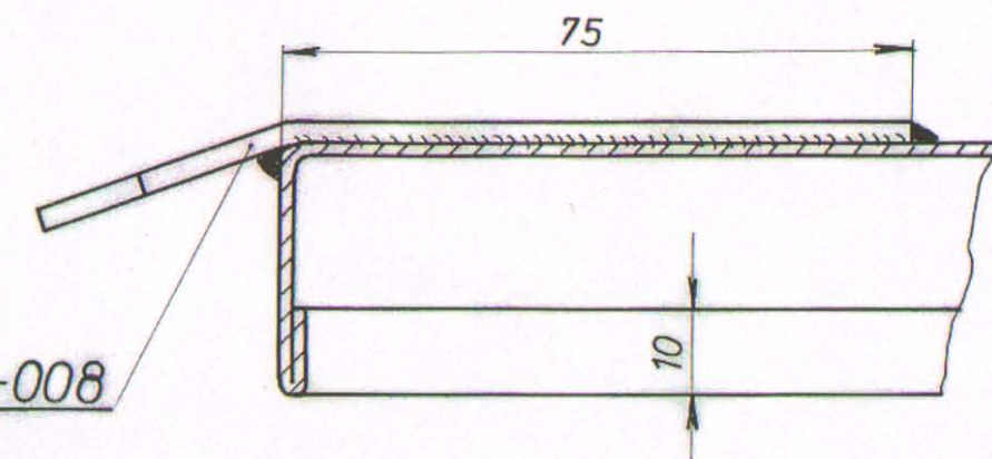
DETALJ „C“ R 1:1
