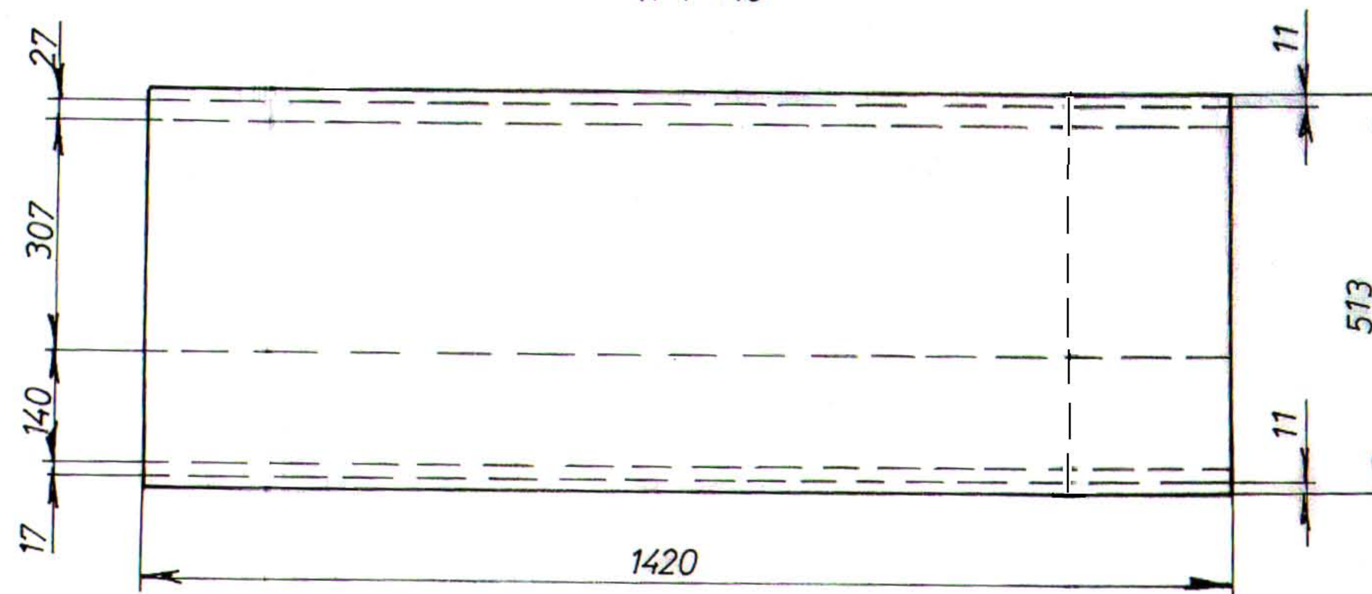
RAZVIJEN OBLIK R 1 : 10
