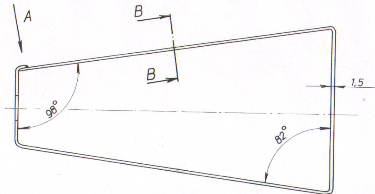
IZGLED OMOTAČA POSLE SAVIJANJA
