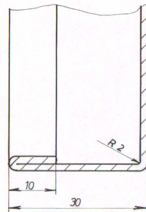
DETALJ „C” R 2:1
