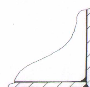
DETALJ „C” R 2:1
