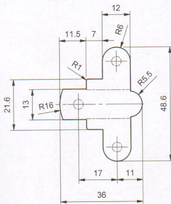
RAZVIJENI OBLIK (R 1:1)
