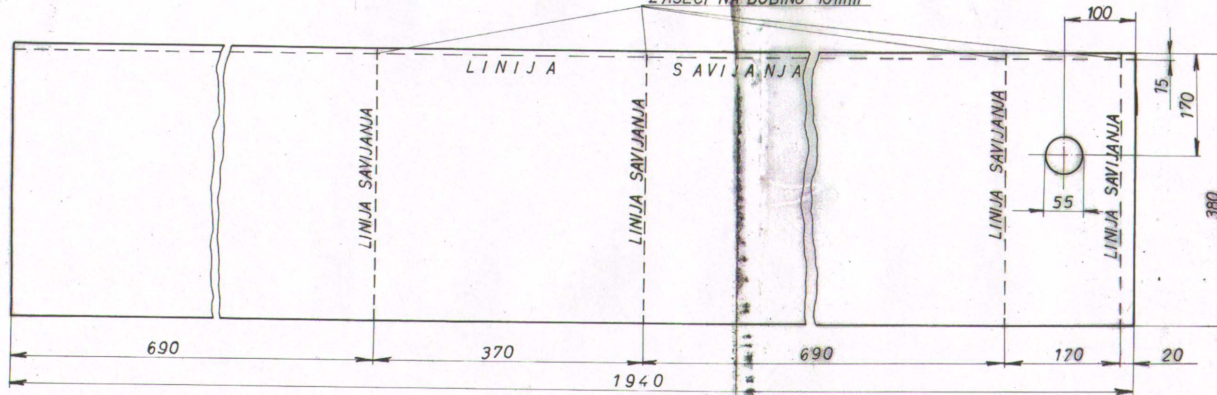
IZGLED OMOTAČA POSLE SAVIJANJA
