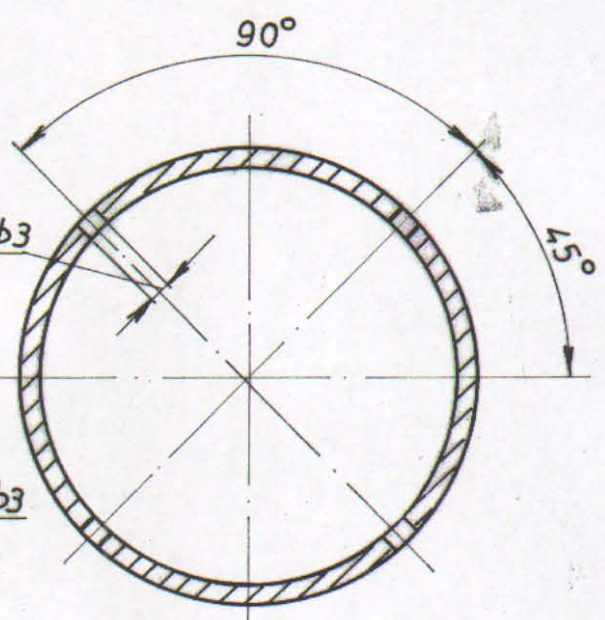
PRESEK B-B
