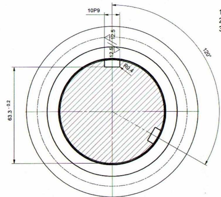
A-A (1:1)
