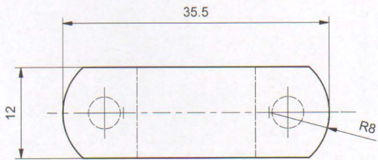
RAZVIJENI OBLIK (R 2:1)
