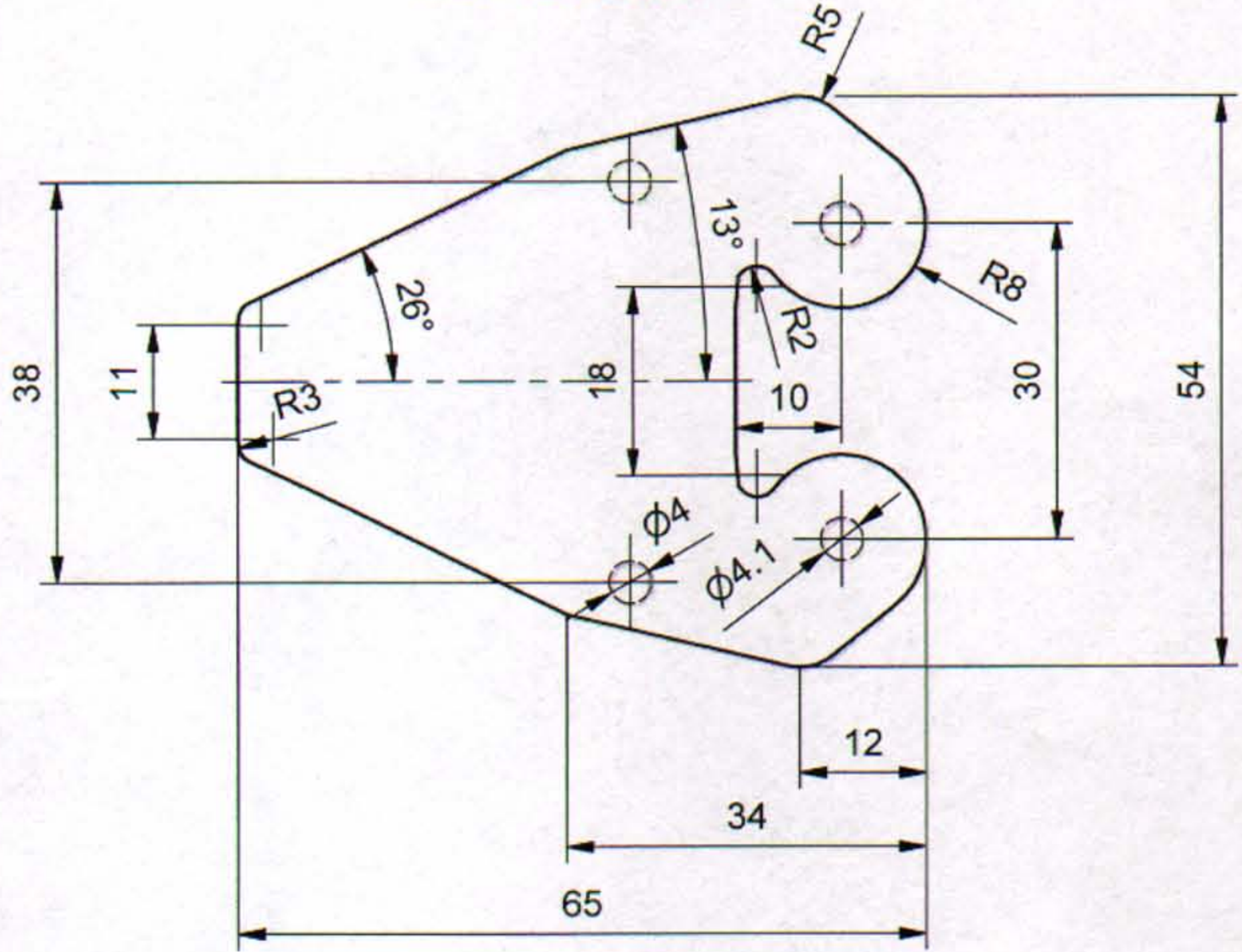
RAZVIJENI OBLIK (R 1:1)
