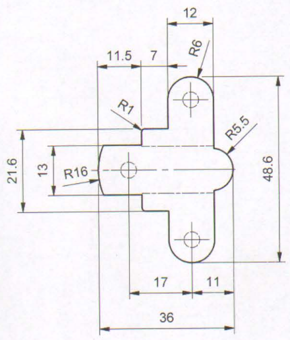
RAZVIJENI OBLIK (R 1:1)
