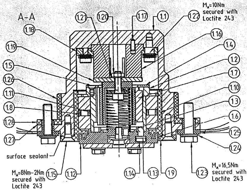
Цртеж склопа осовинског уземљења CAF са деловима:
